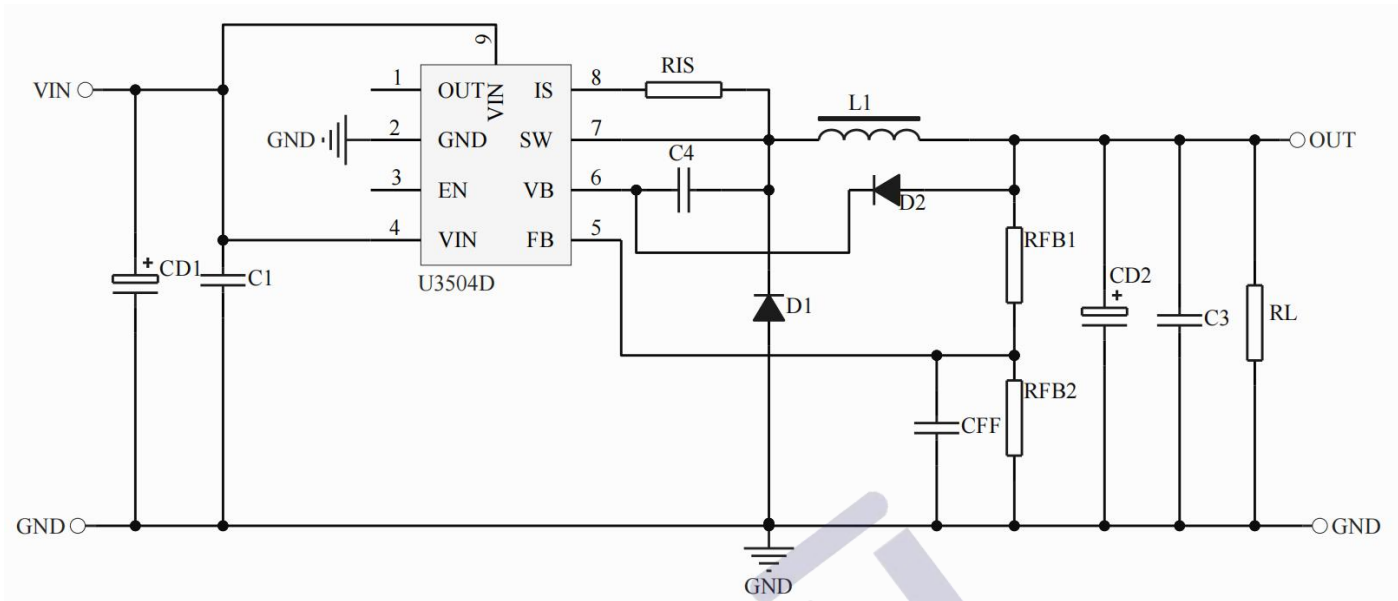
APP3:VOUT=10~15V
